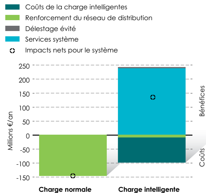
Graphique 2 Coûts et bénéfices de l'intégration des véhicules rechargeables dans les réseaux de distribution d'électricité en France. Source : Element Energy
